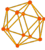
Ikosaeder
