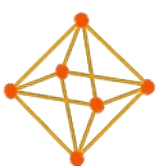
Oktaeder
