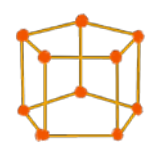
Fünfseitiges Prisma
